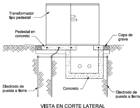
Figura 8. Sistema puesta a tierra.
